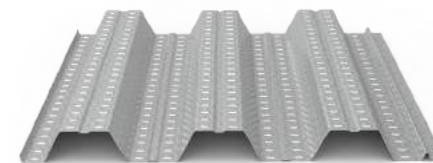
Tôn sàn 3 sóng H50 - W1000 H50 - W1000 3 square decking panel
